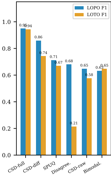
F1 Score
