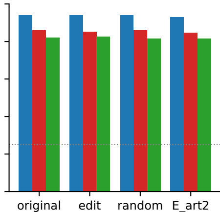
Gemma-3-12B-IT
