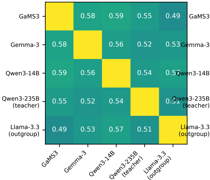
HARD-DEV EN original (n=487)
