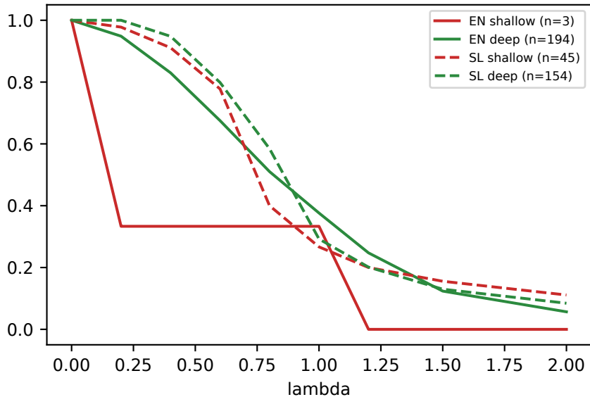
Gemma-3-12B-IT
