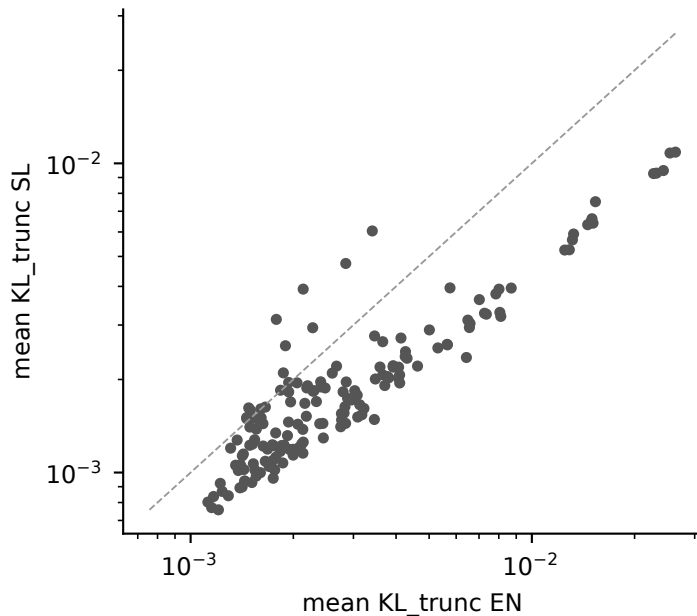
per-edit divergence, EN vs SL (F)
