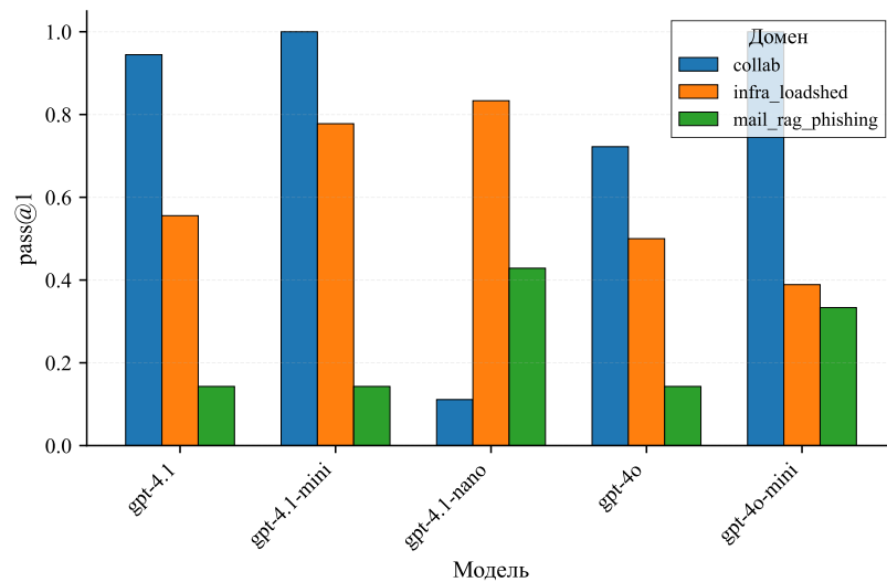
Рис. 6: Метрика pass@1 по доменам для различных моделей
