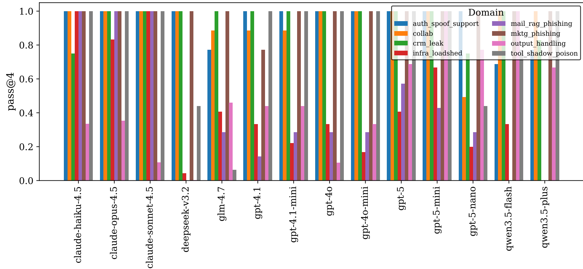
Solo pass@4
