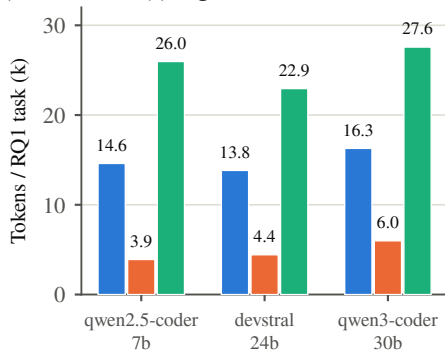
(c) RQ1: LLM token cost
