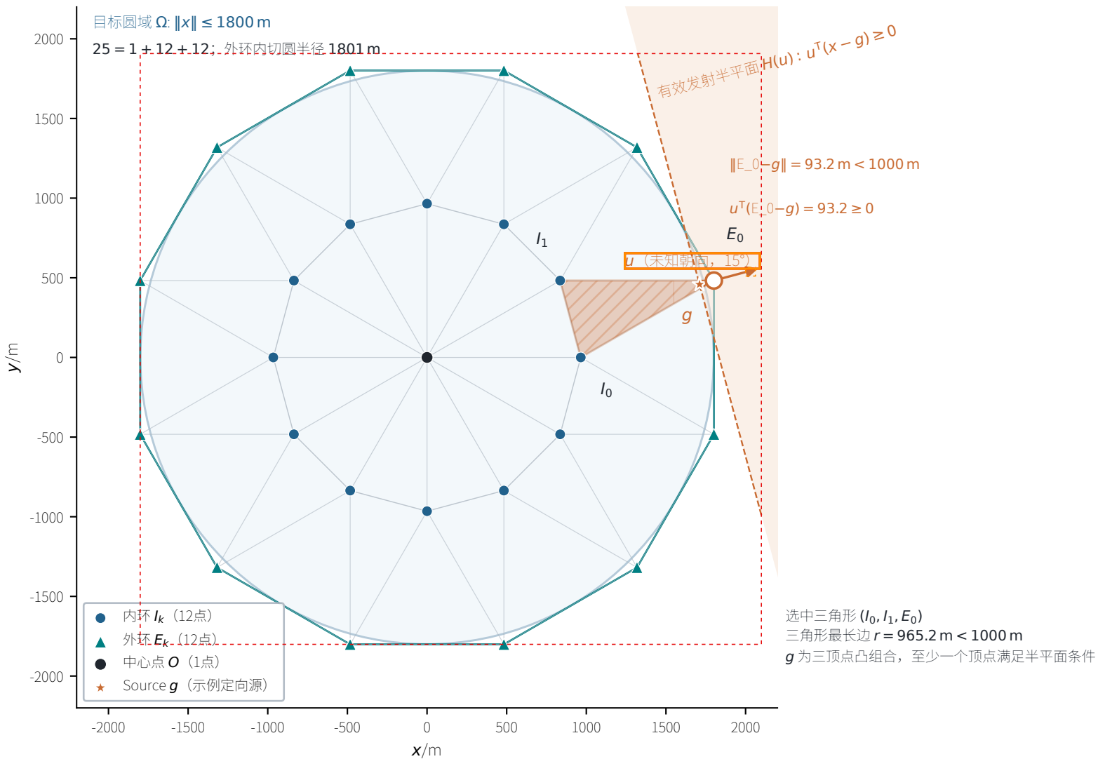
问题四内外联合网格及定向干扰源发现覆盖示意图
