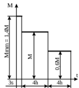
Đặc tính tải trọng
