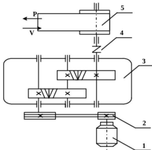
Sơ đồ động của hệ thống
