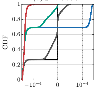
(d) S2 violation
