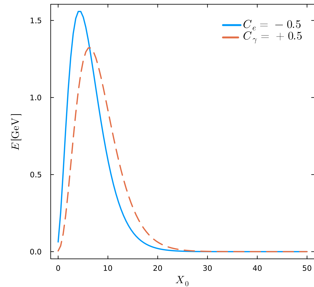
E = 25.0 GeV
