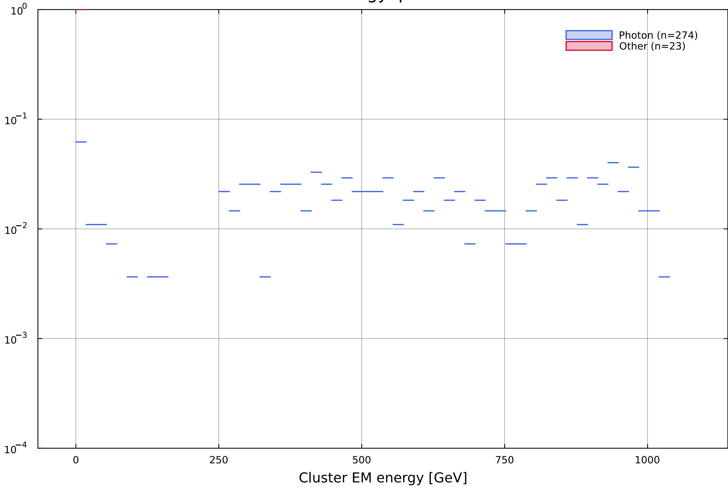
Cluster EM energy: photon vs other
