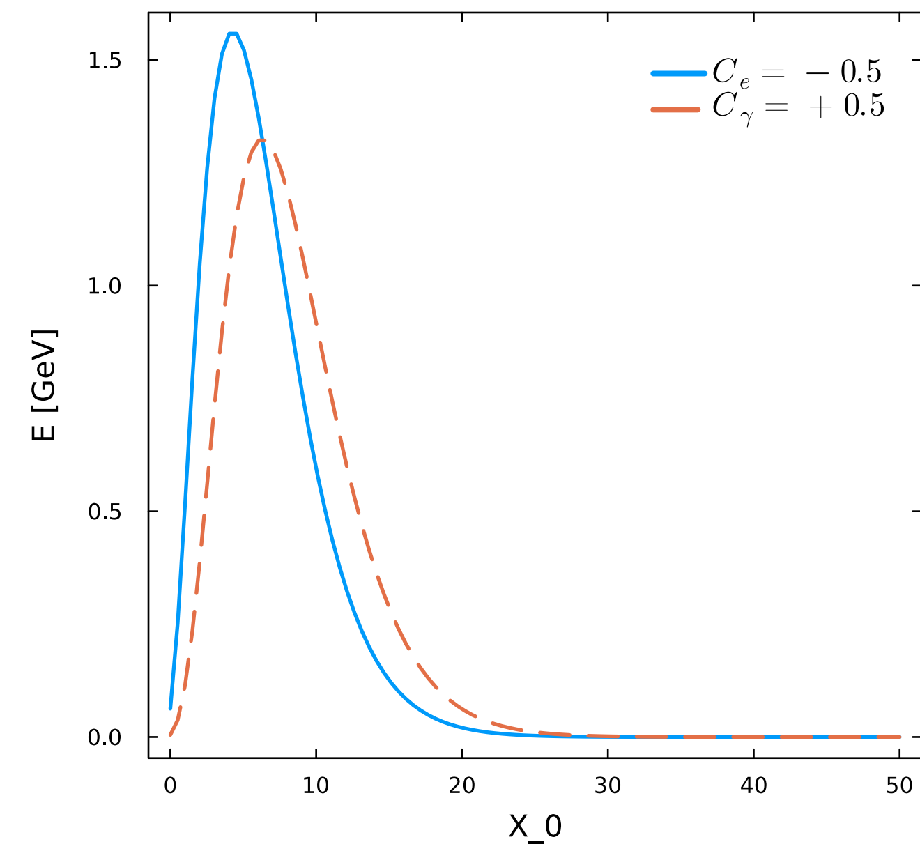
E = 25.0 GeV
