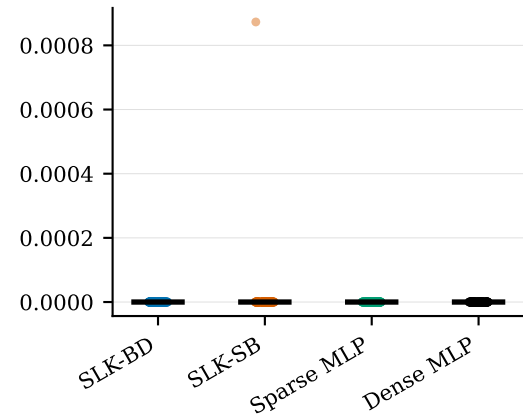
H(B | S) deep
