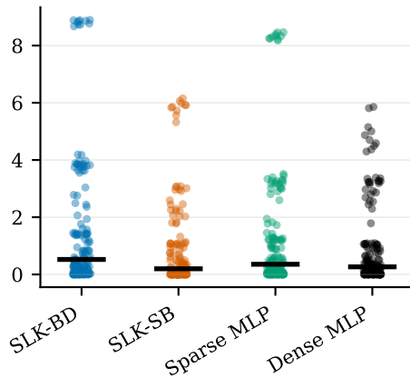
H(S | B) deep
