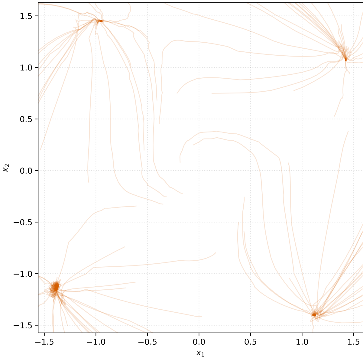
var_depth_gradient_4
