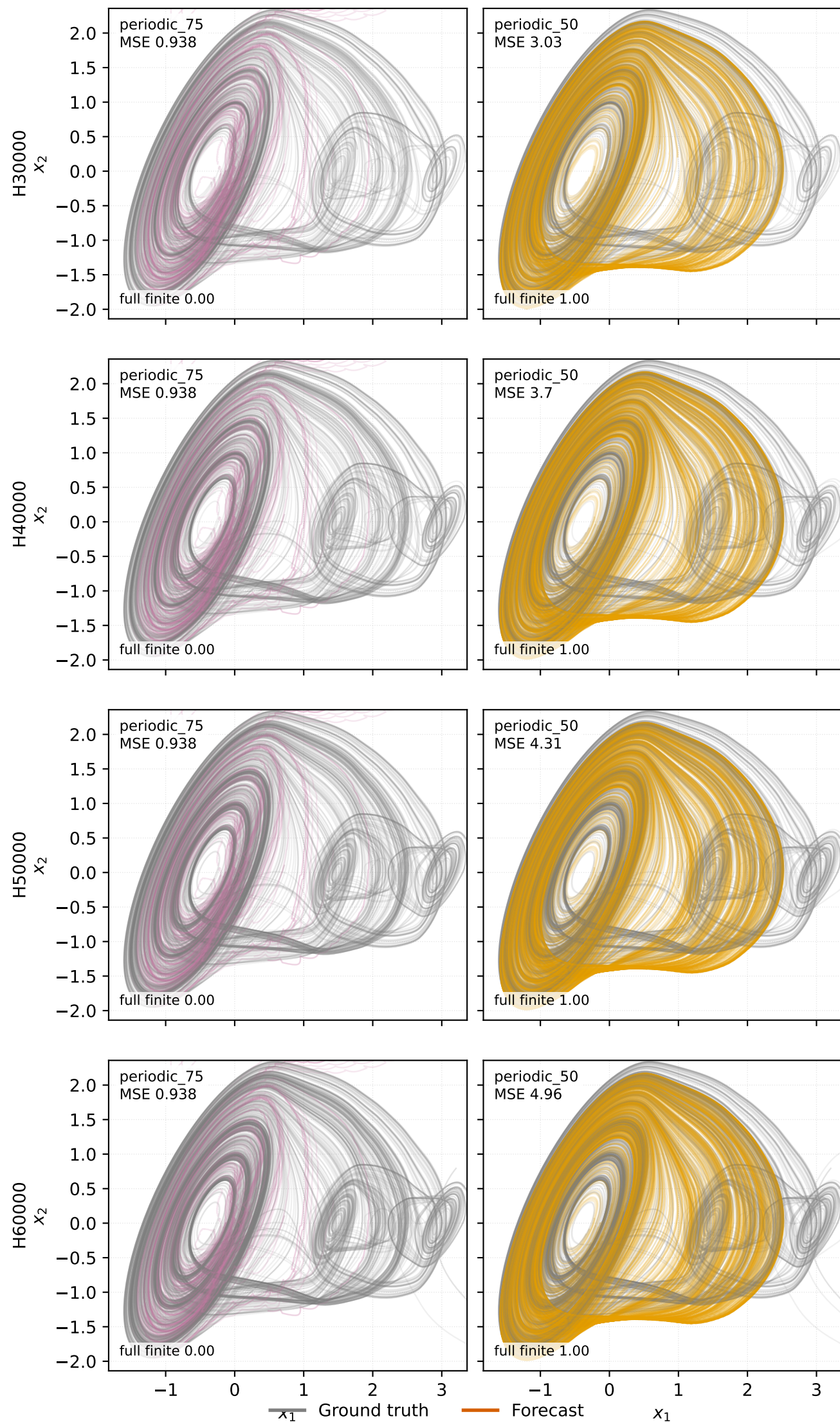
LISTA-BD
