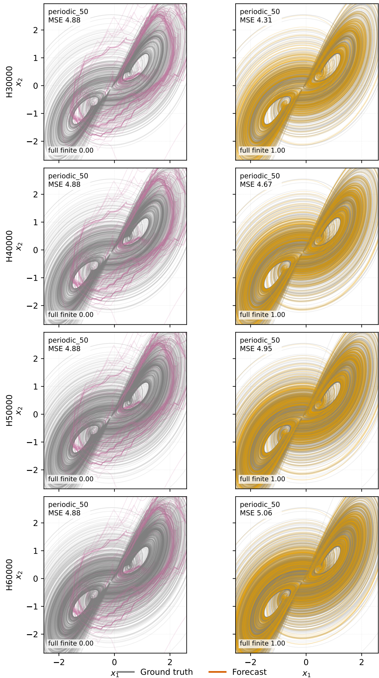
LISTA-BD
