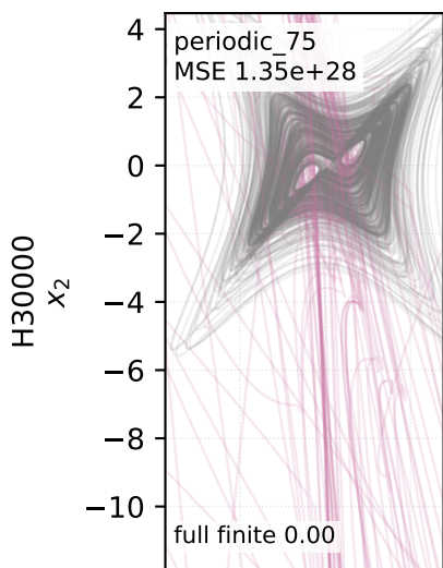
LISTA-BD
