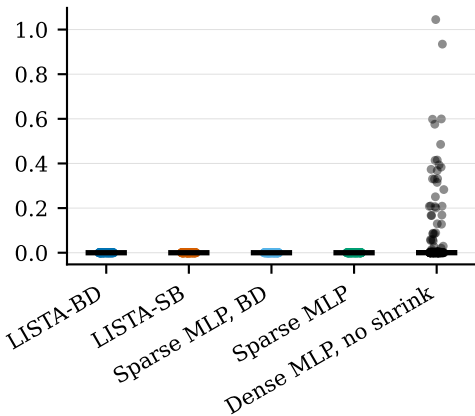
H(B | S_{\text{abs}})
