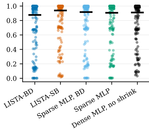
U_{\text{exact}} deep
