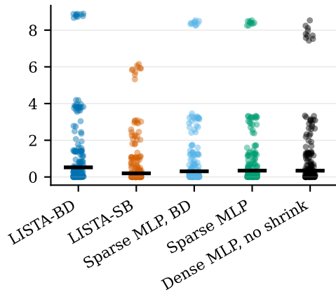
H(S|B) deep
