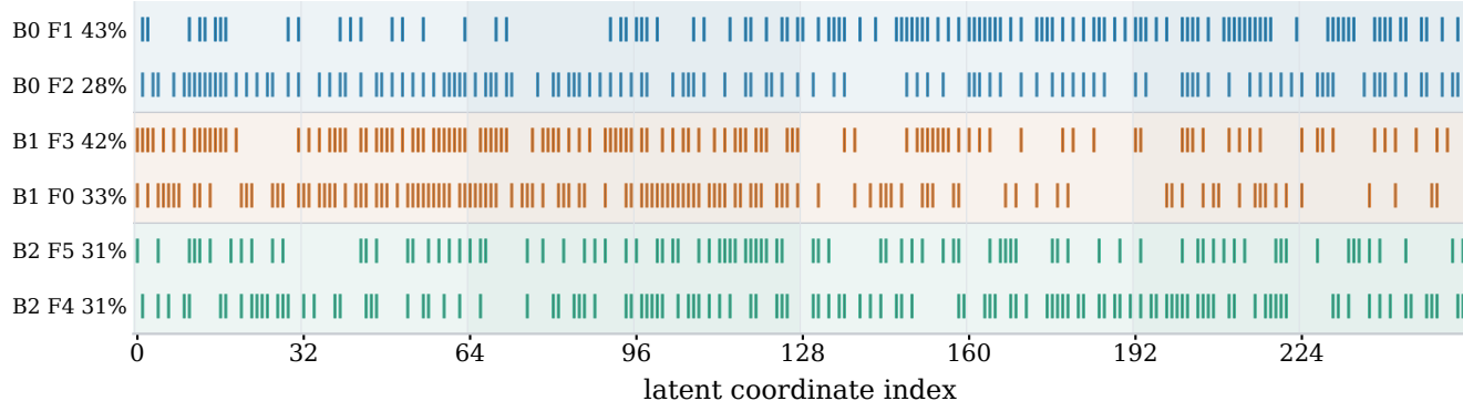
LISTA-BD | Local-linear gates | F_abs
