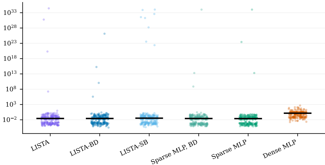
H1000 MSE per dimension
