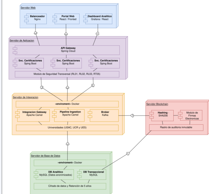
DIAGRAMA DE DESPLIEGUE
