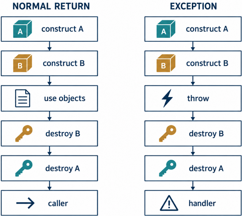
图 4.1 正常返回与异常传播都利用对象销毁完成清理。这里假设两个局部对象均已成功构造，异常被外层处理器接住。
