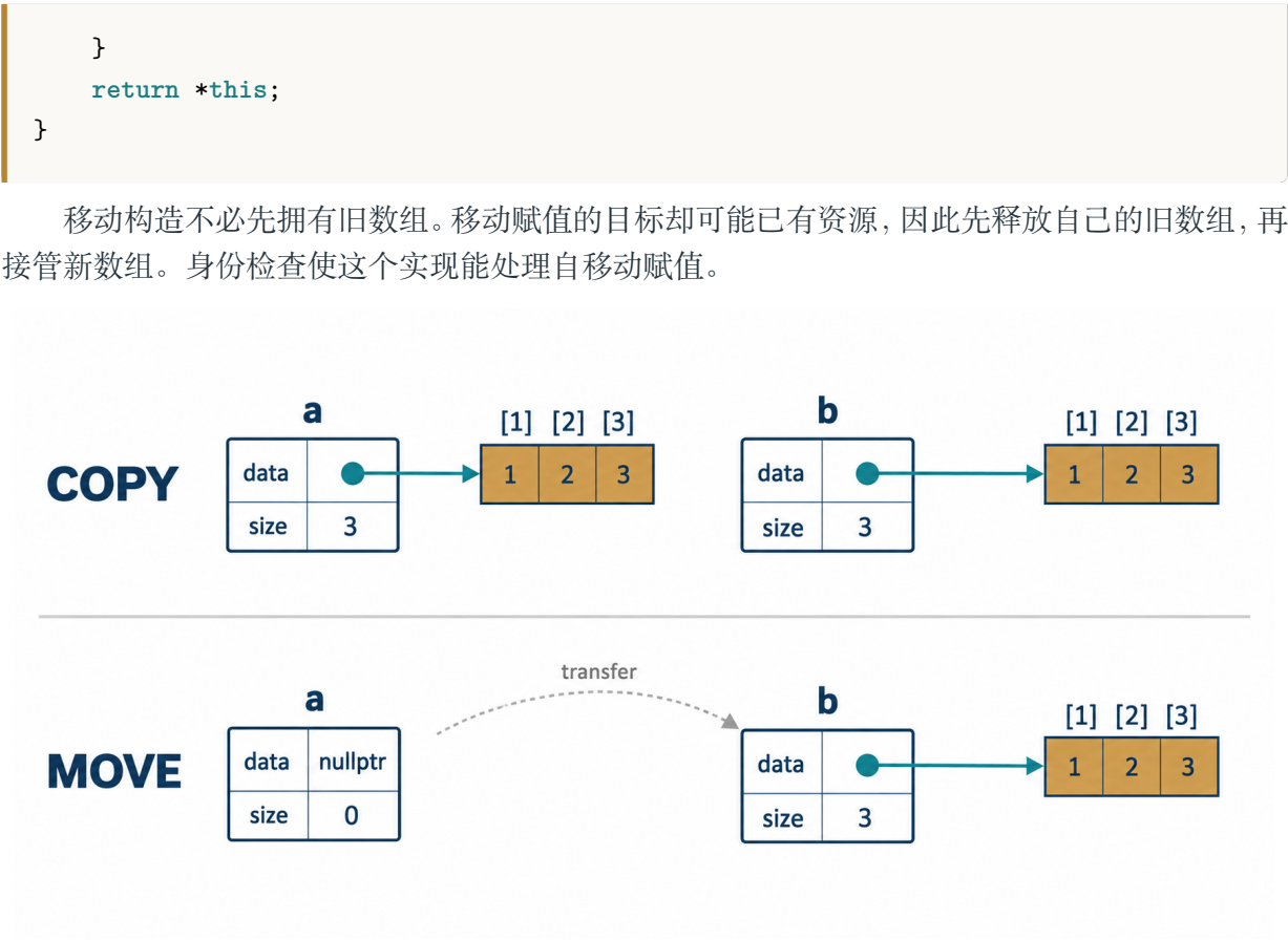
图 8.1 教学 Buffer 的复制与移动结果。复制建立独立数组，移动转交已有数组。方格中的 1、2、3 表示数据内容；源对象变空是本类的明确约定。
