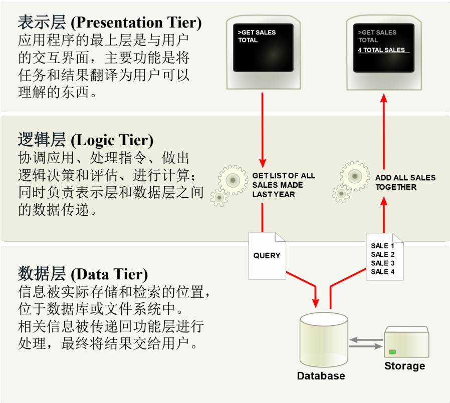
图 14.1 表示、业务逻辑与数据层是一种常见分工。箭头与边界应反映实际职责；把类放进三个文件夹，并不会自动得到良好分层。（课程第 14 讲，第 16 页）
