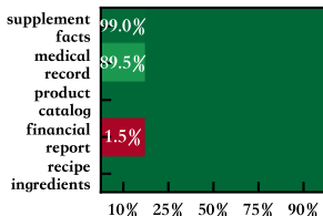
B3 jsonrepair
