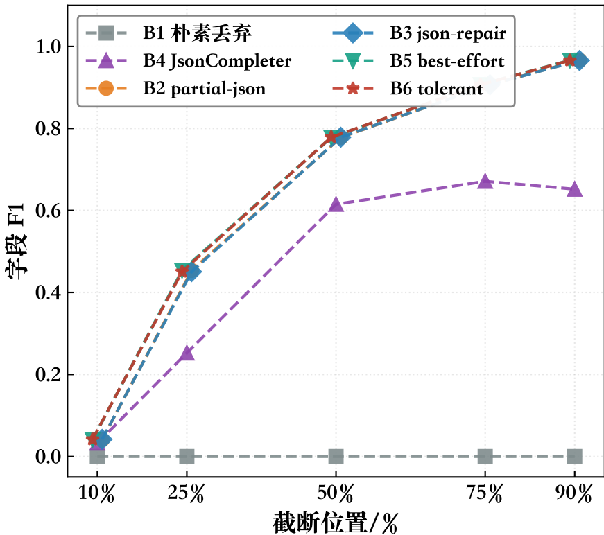
各方法字段 F1 随截断位置的变化
