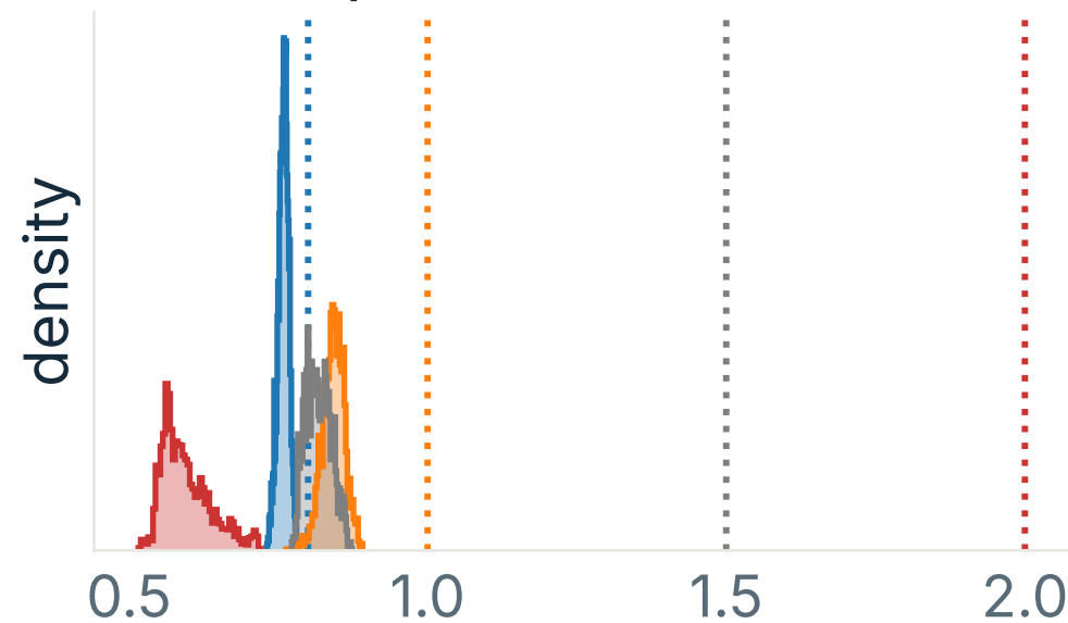
posterior of W
