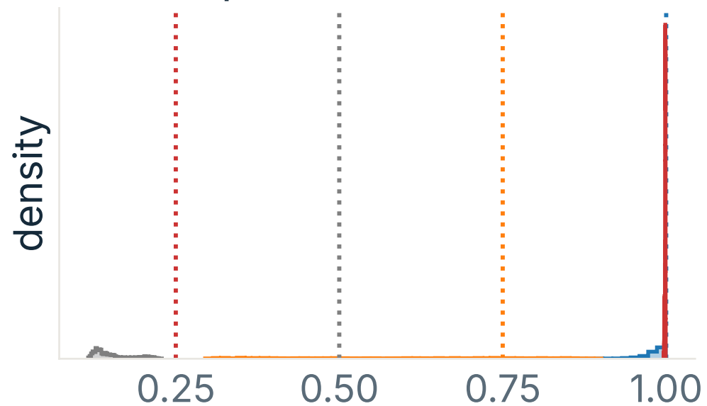
posterior of \theta_P
