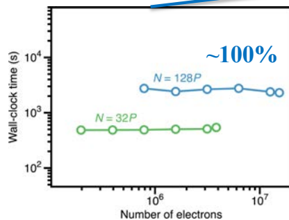
DC-MESH NAQMD
