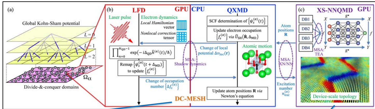
DC-MESH NAQMD
