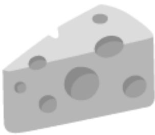
QUESO
