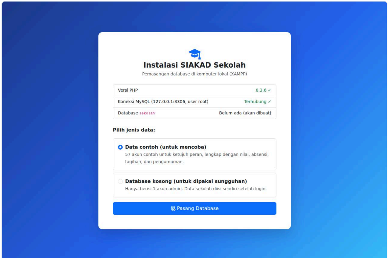
Halaman instalasi otomatis
