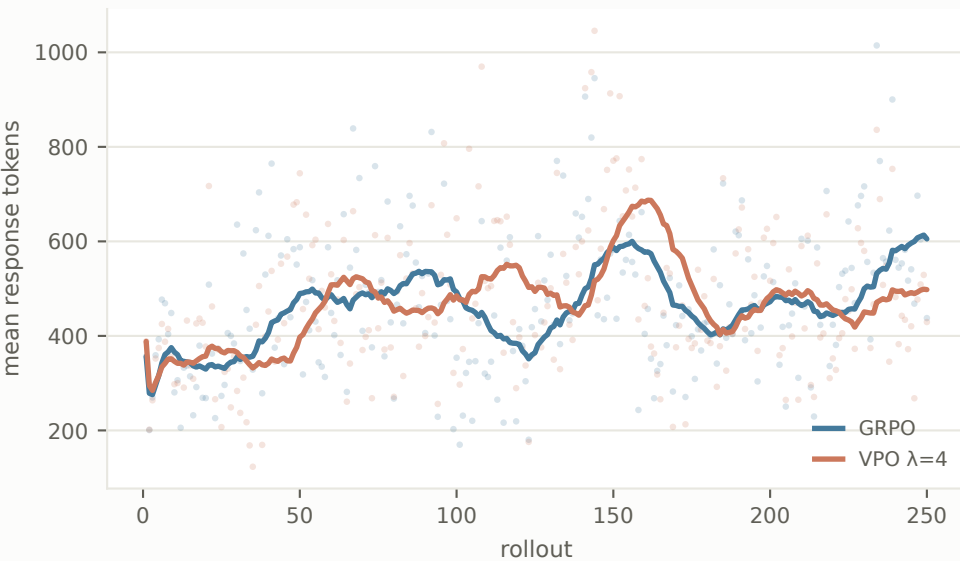
Llama-3.1-8B Base → SFT → RL
