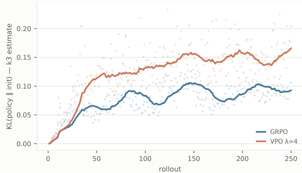
Llama-3.1-8B Base → SFT → RL
