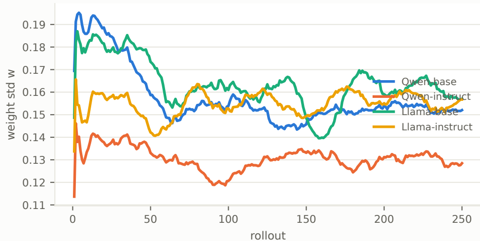
VPO \lambda=4 : weight std w
