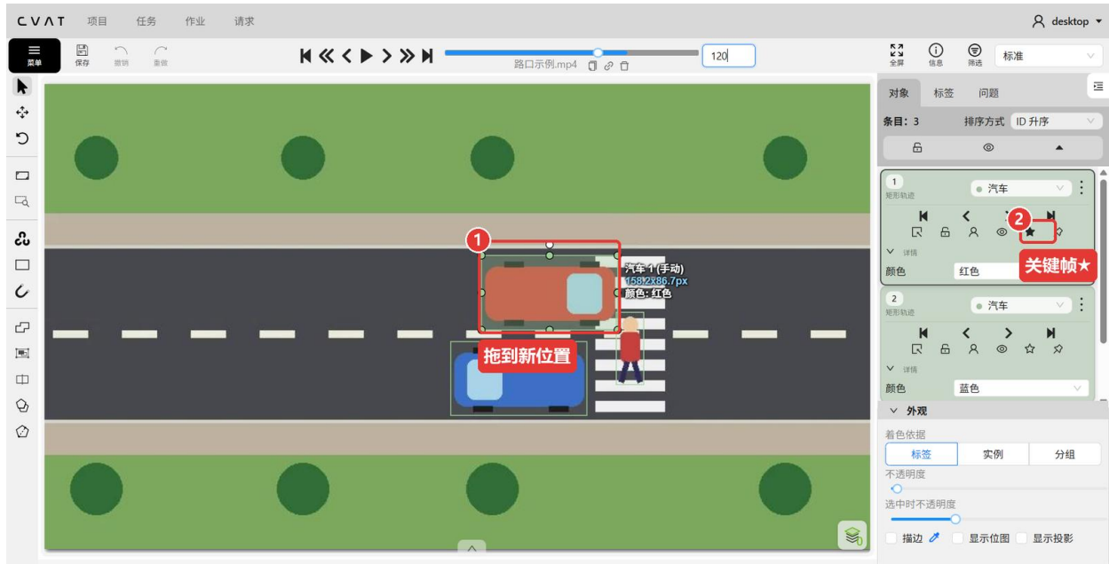
图 12 在第 120 帧调整位置，自动生成关键帧
