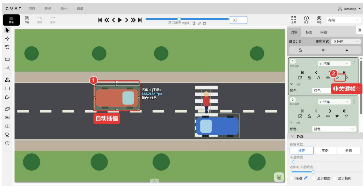
图 13 第 80 帧由关键帧自动插值
