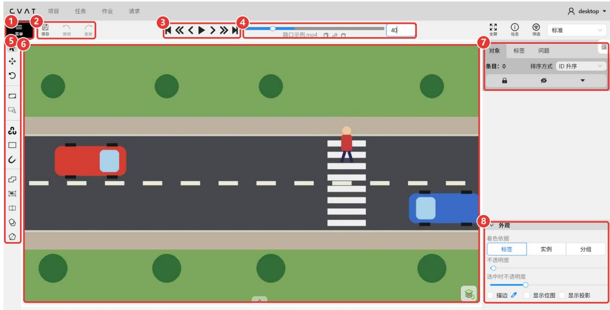
图 7 标注工作区（编号对应下表）
