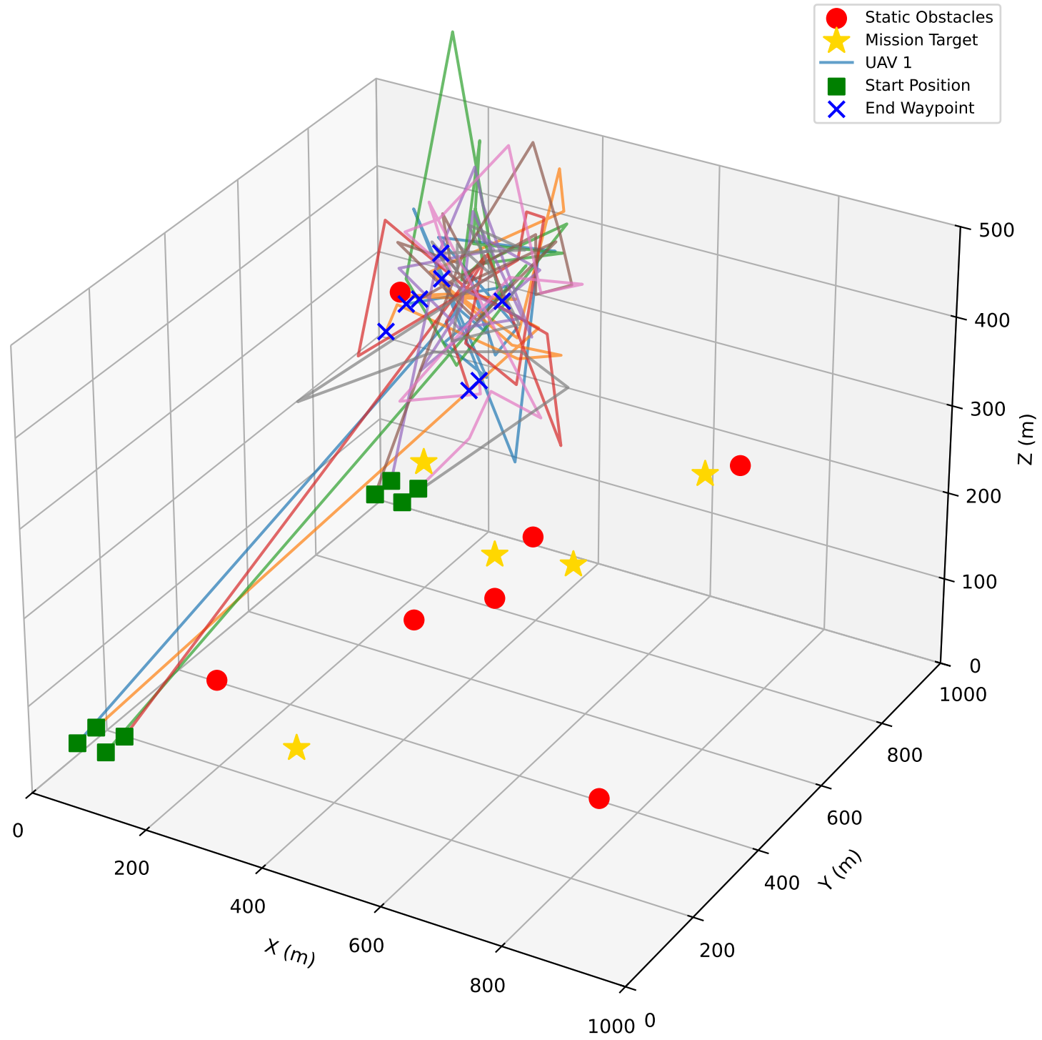
QISO Optimized Paths - Scenario_2_QISO_DynamicW
