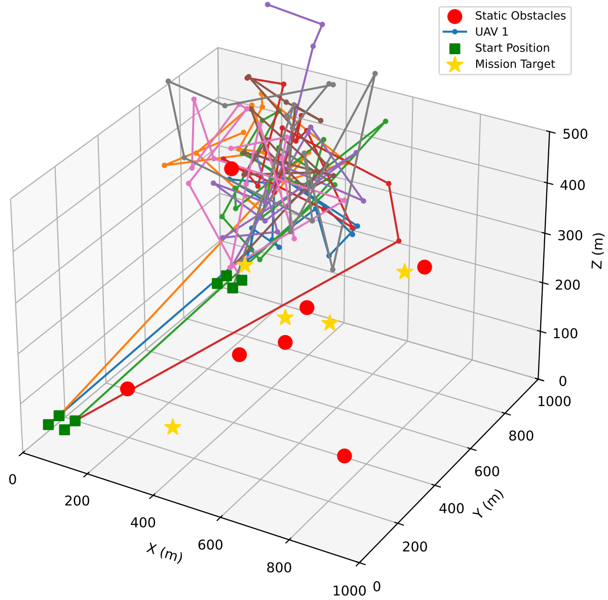
QISO Optimized Paths - Scenario_2_QISO
