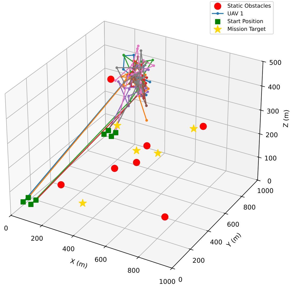
SPSO Optimized Paths - Scenario_2_Baseline
