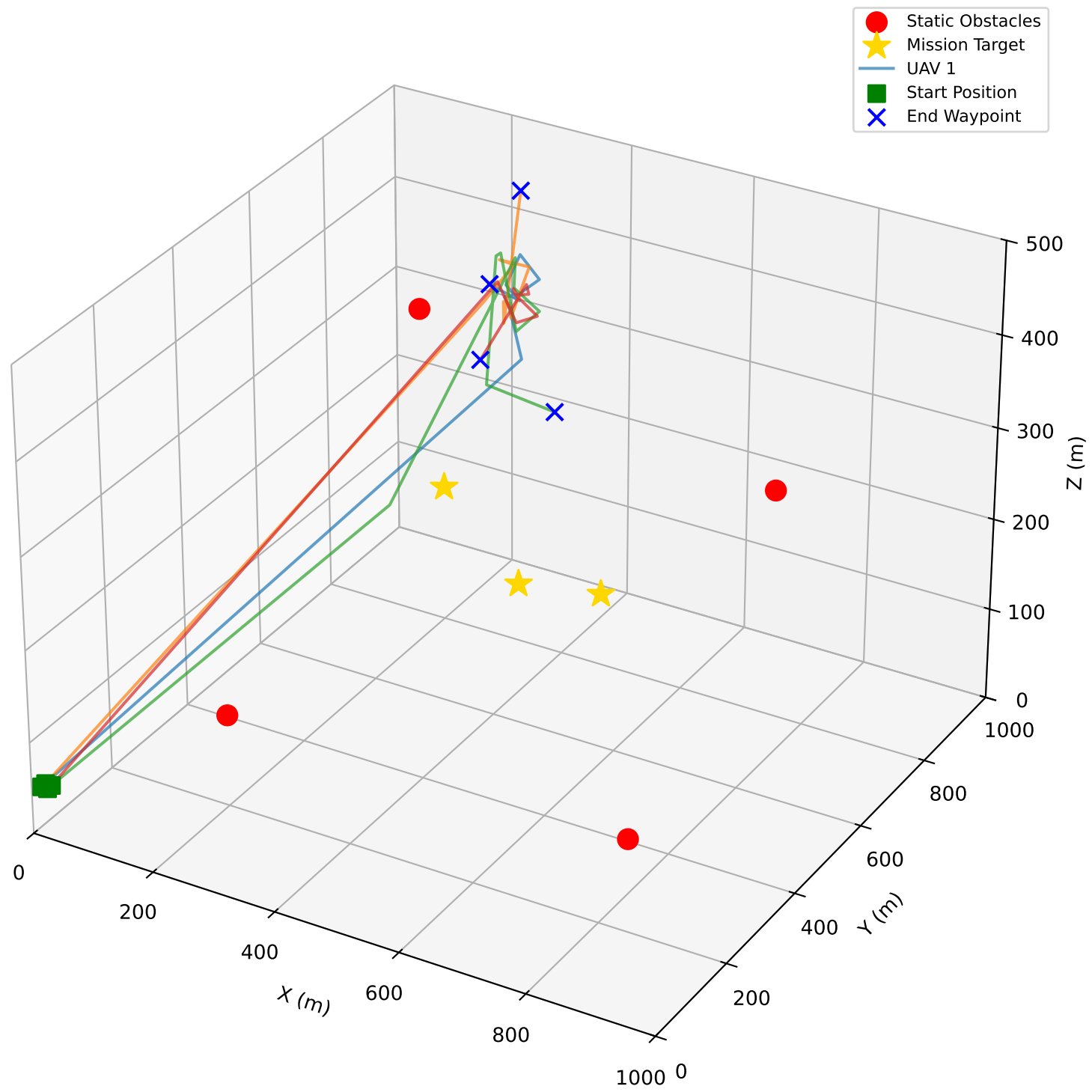
SPSO Optimized Paths - Scenario_1
