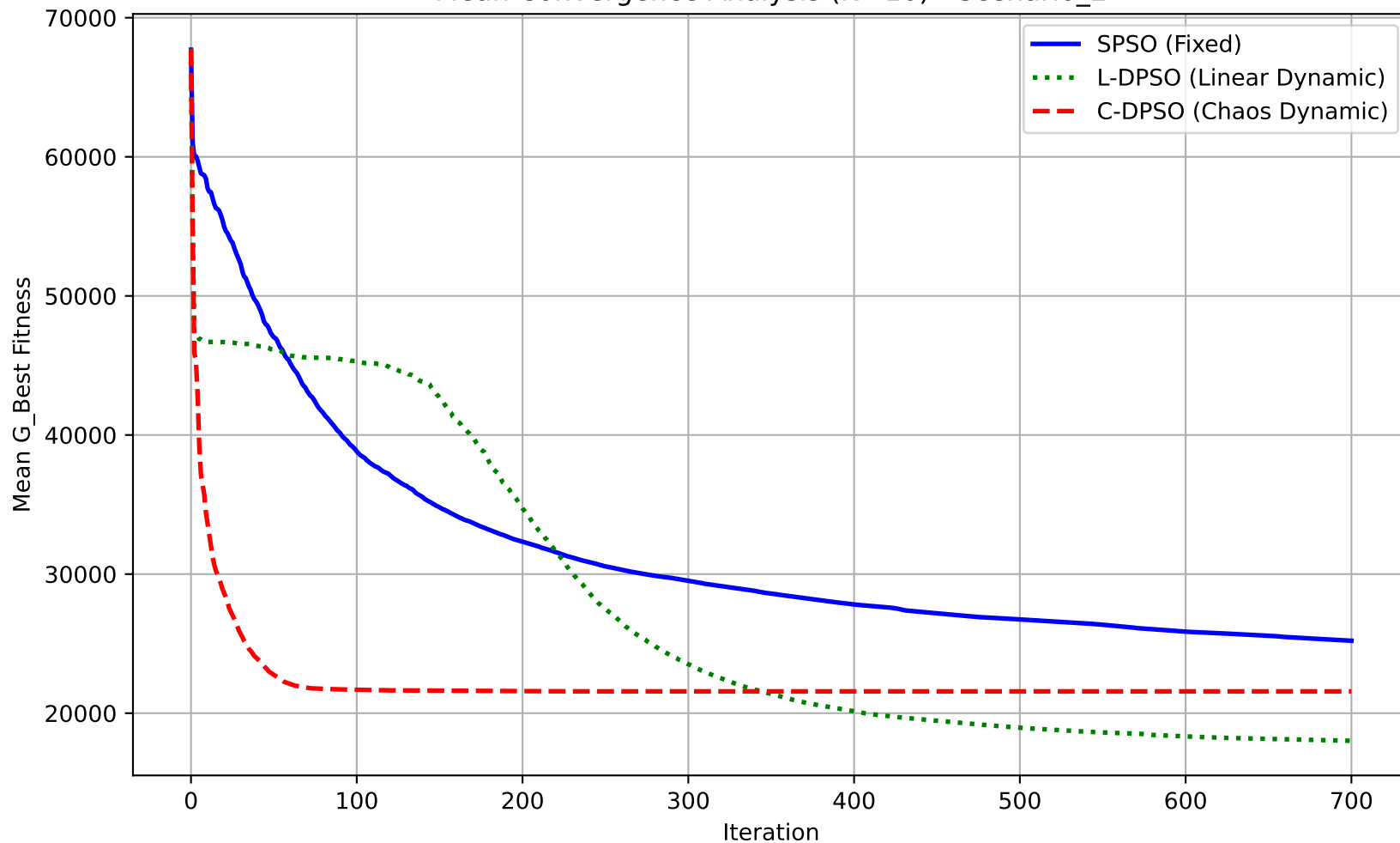
Mean Convergence Analysis (N=10) - Scenario_2
