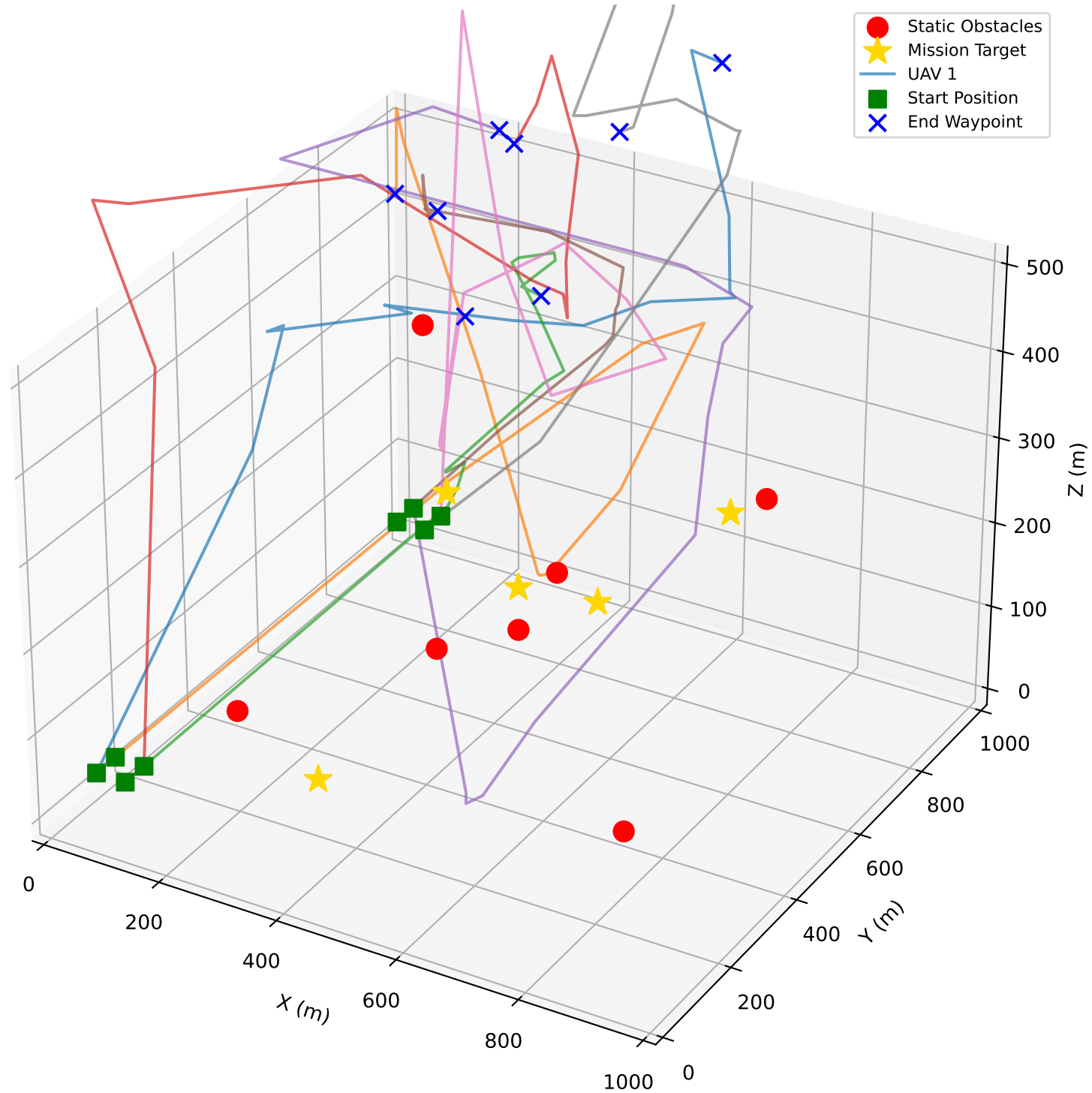
L-DPSO Optimized Paths - Scenario_2_LDP
