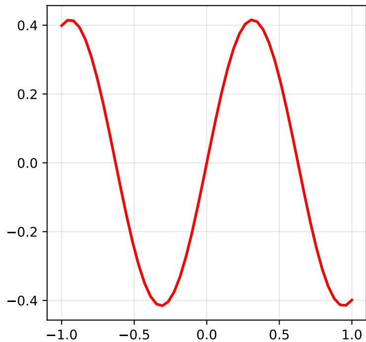
Latent Dim 51
