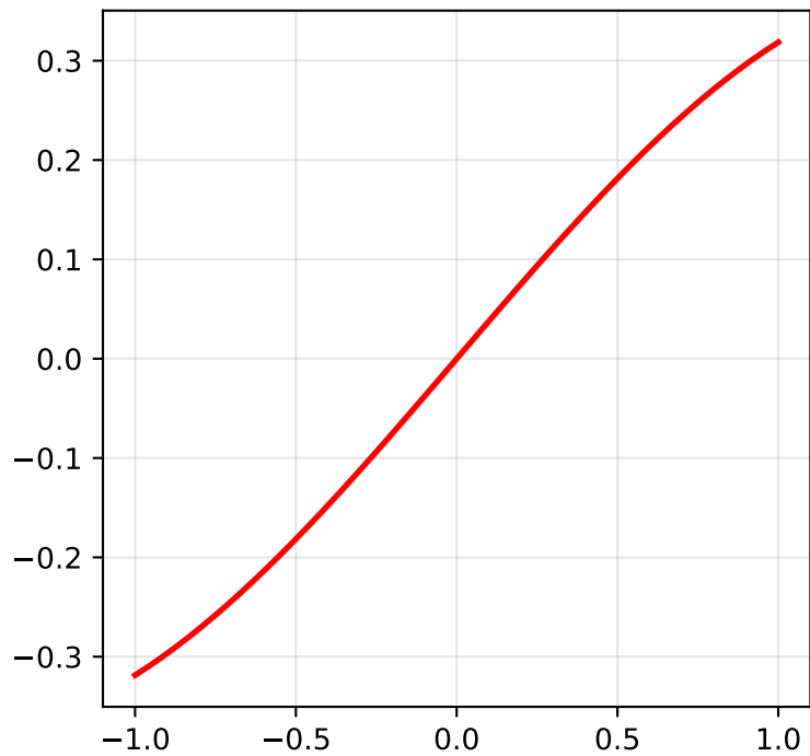
Latent Dim 63
