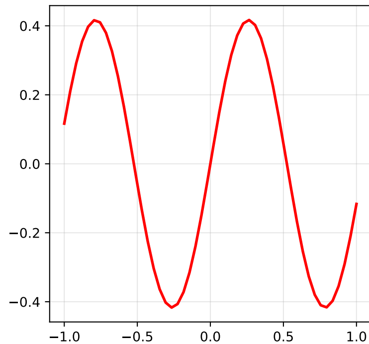
Latent Dim 59
