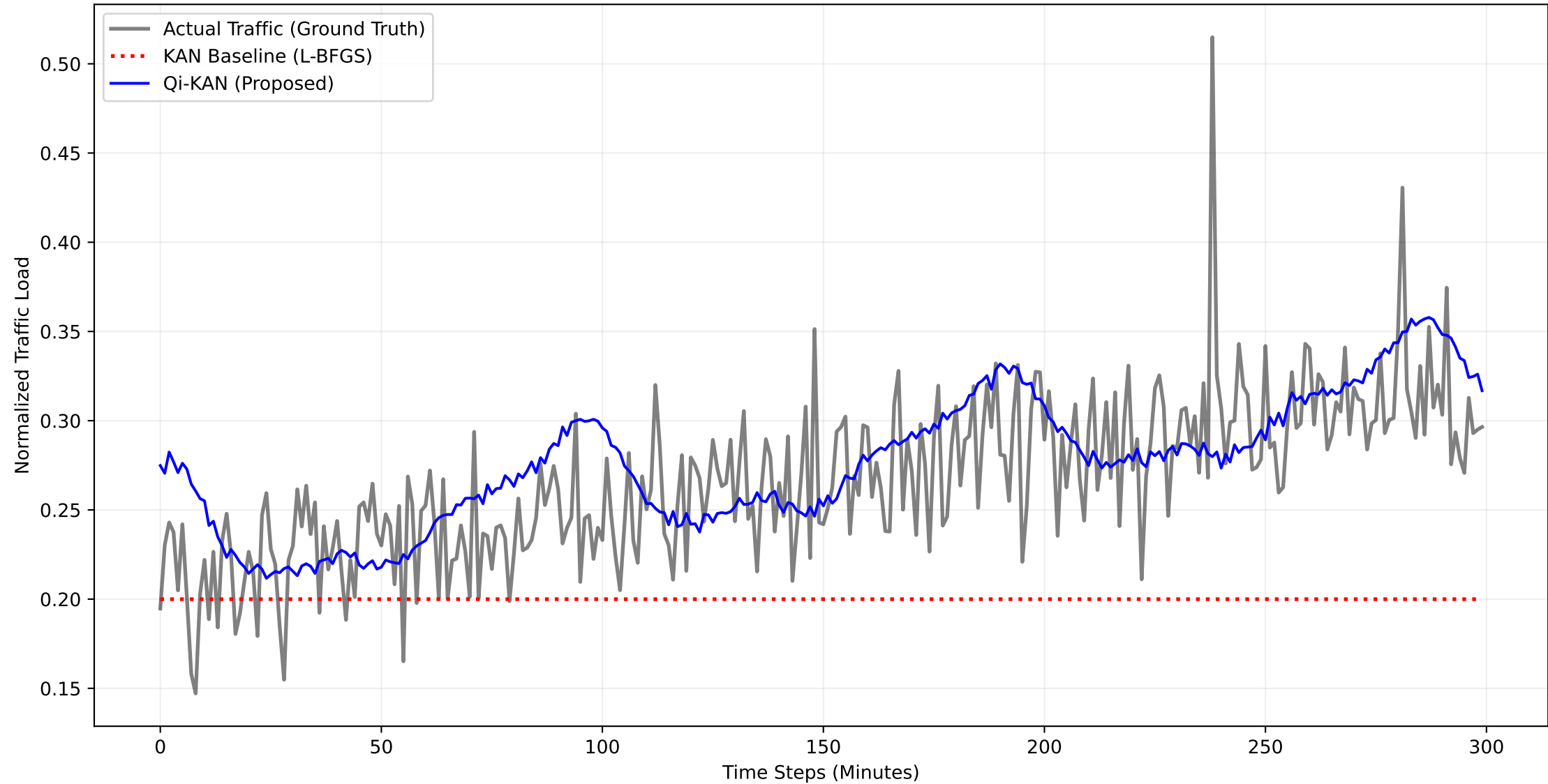
Performance Comparison: KAN vs Qi-KAN (Urban Scenario)
