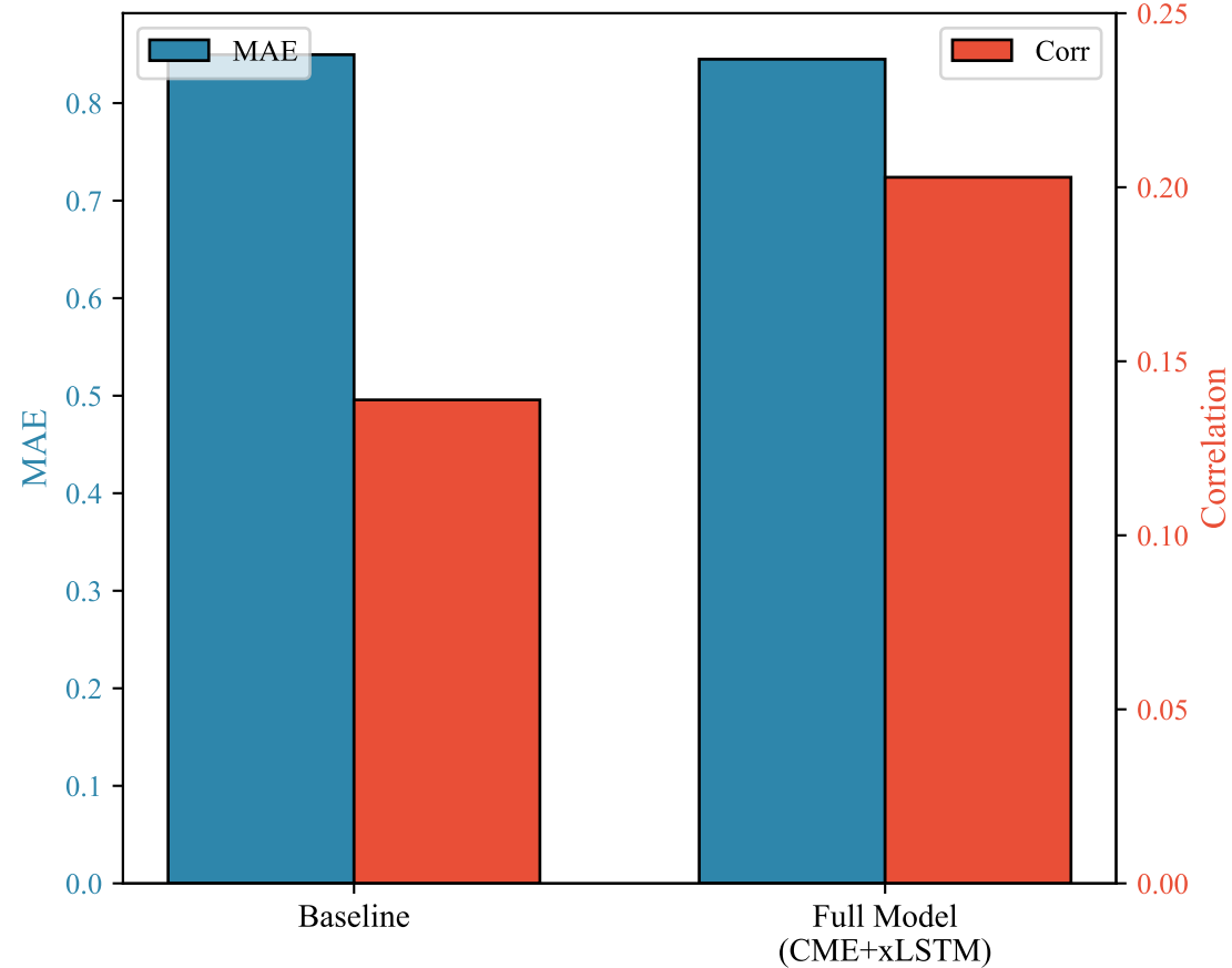
MOSEI: xLSTM Contribution
