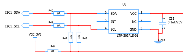
环境光传感器
