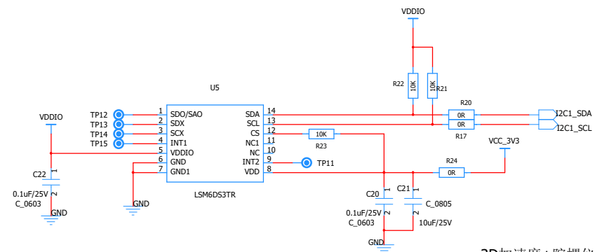
3D加速度+陀螺仪
