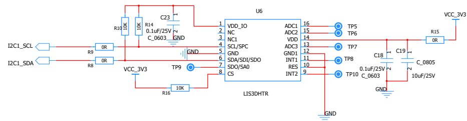
3D加速度计
