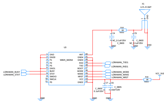
LORAWAN 模块 868 (兼容470)
