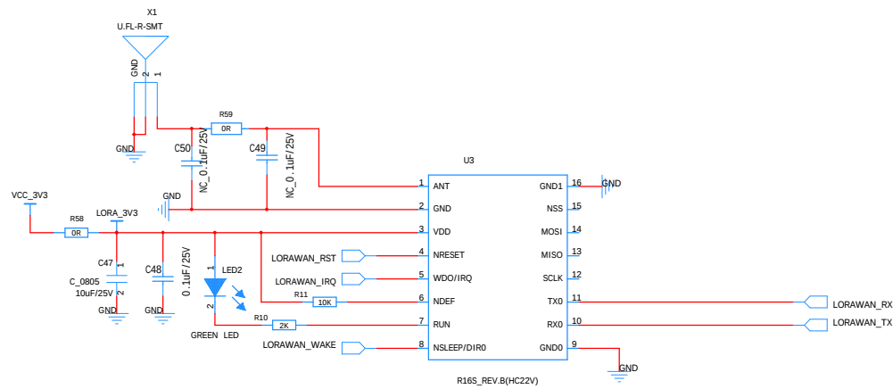
LoRaWAN模组
