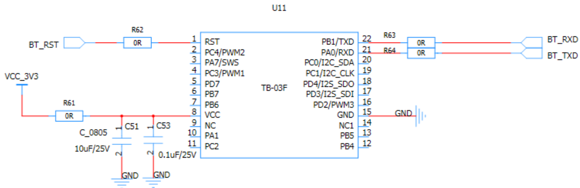
蓝牙模组
