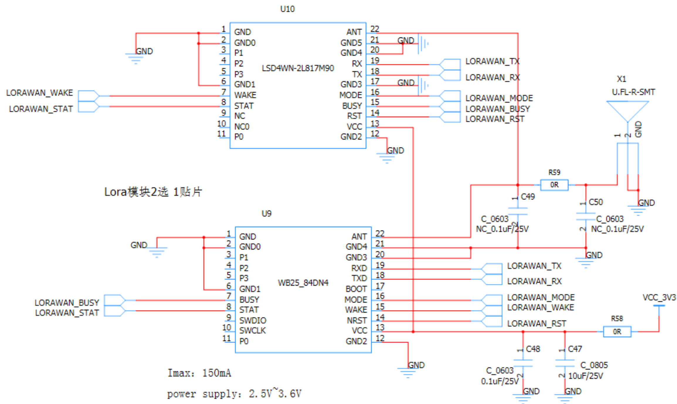
LoRaWAN模组
