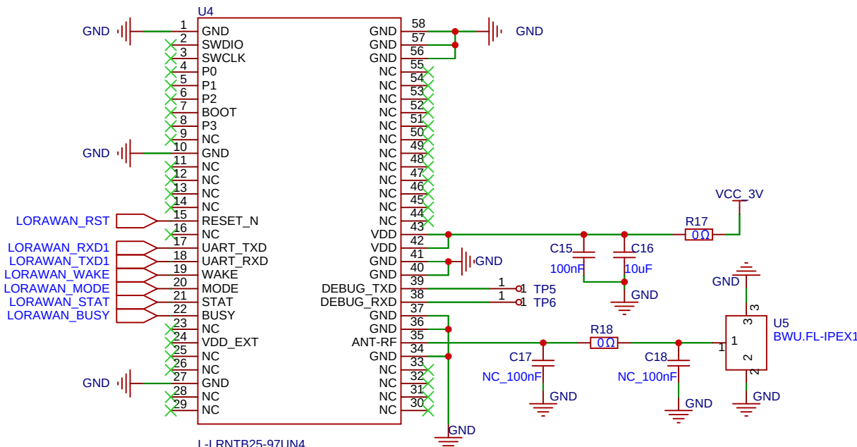
LoRaWAN模块
