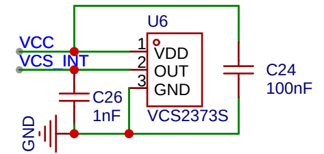
磁开关
