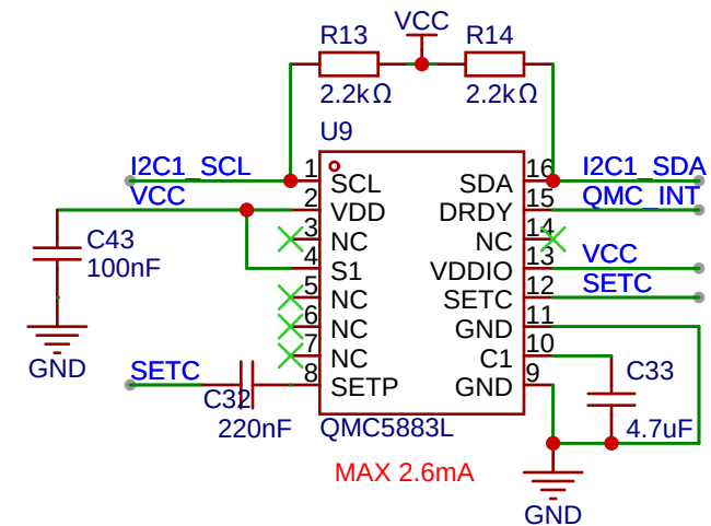
磁力计
