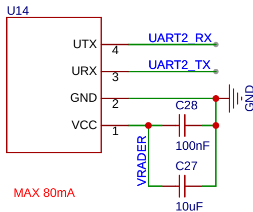
雷达模块
