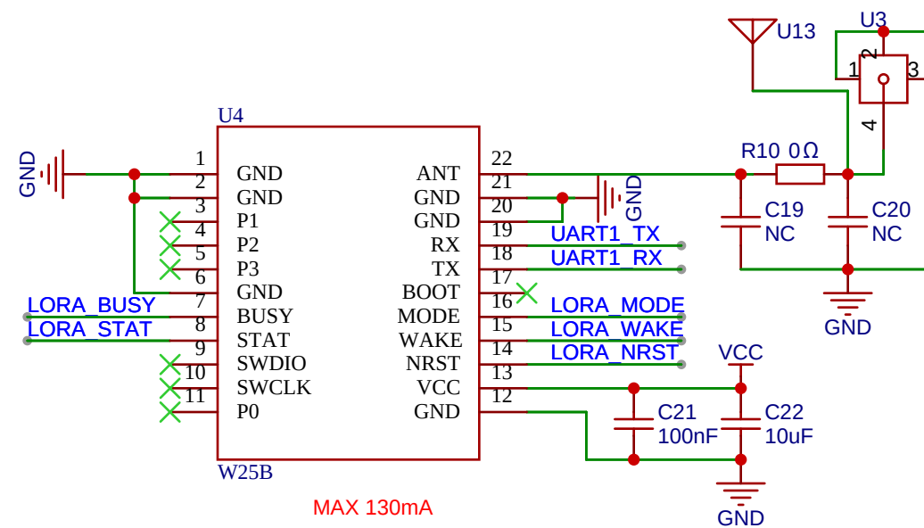
LoRaWAN模块
