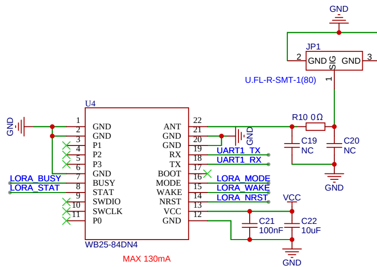
LoRaWAN模块
