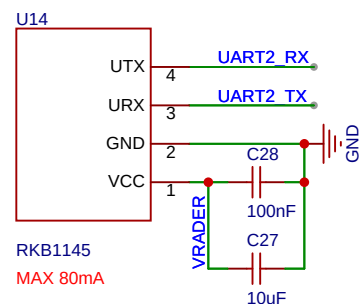
雷达模块
