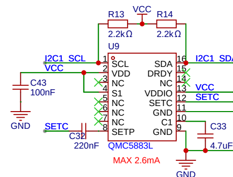
磁力计
