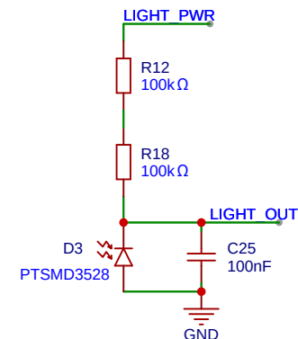
环境光检测/防拆
