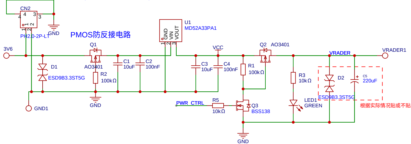
雷达电源控制电路
