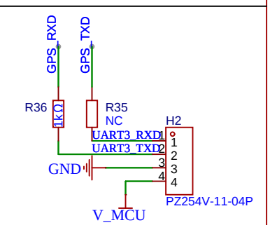
MCU调试口
