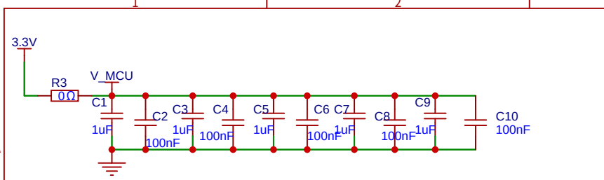
MCU电源
