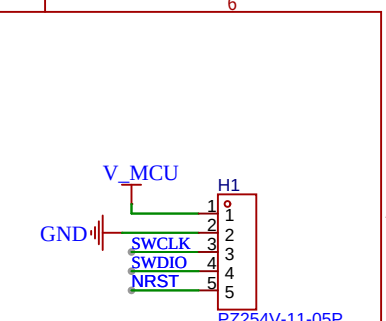
烧录口
