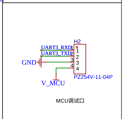
烧录口
