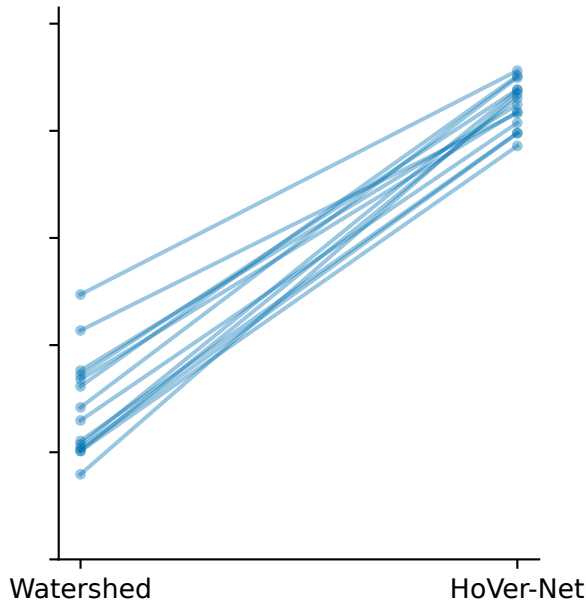
Detection F1
